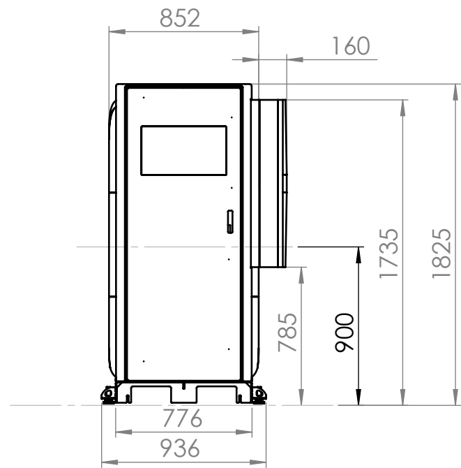
SCALE 1 : 30
