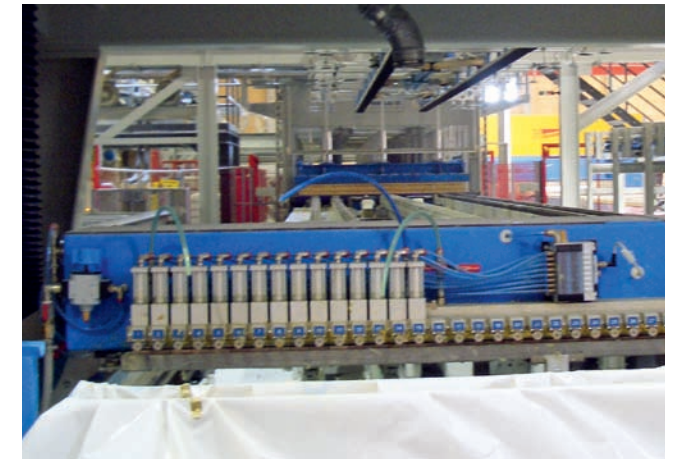
Kleberauftrag Glue Application
