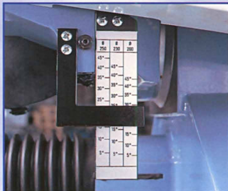
Scala di riferimento per spoglia posteriore Back clearance reference scale Echale de référence pour la dépouille postérieur Masstab für Winkel hinten
