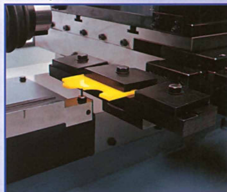
Dima e tastatore Template and stylus Gabarit et doight de copiage Schablone und Taster
