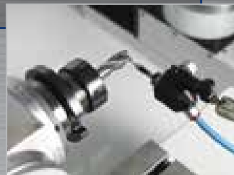
Taster zur Erfassung der Schraube und andere Werkzeugparameter. Probe to teach-in the helix and other tool parameters.
