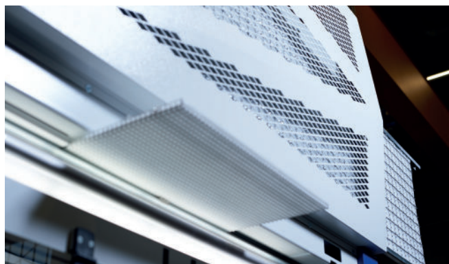
Alle Filter sind mit einem Schnellwechselsystem ausgestattet. 5 Filterebenen sorgen für optimale Umgebungsluft in der Lackierkabine.
